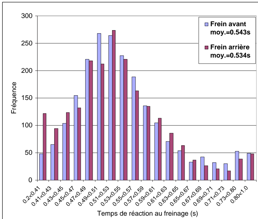
Figure 6 □ Fréquence obtenue en fonction du temps de réaction au freinage en procédure non couverte, pour les hommes.
