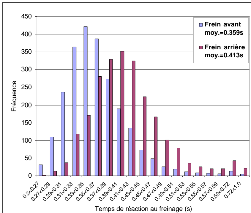
Figure 9 □ Fréquence obtenue en fonction du temps de réaction au freinage en procédure couverte, pour le groupe mixte comportant les femmes et les hommes.
