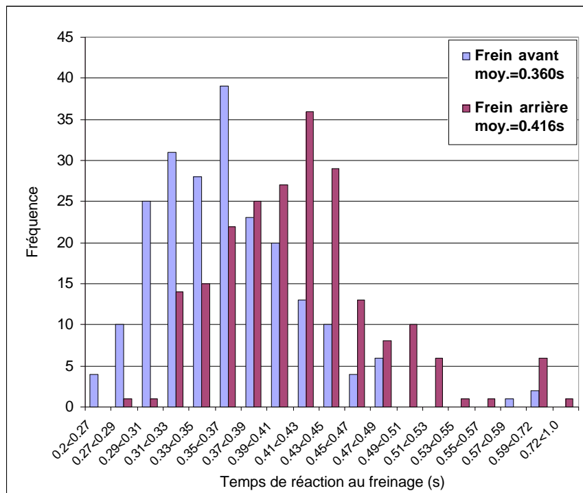
Figure 5 □ Fréquence obtenue en fonction du temps de réaction au freinage en procédure couverte, pour les femmes.
